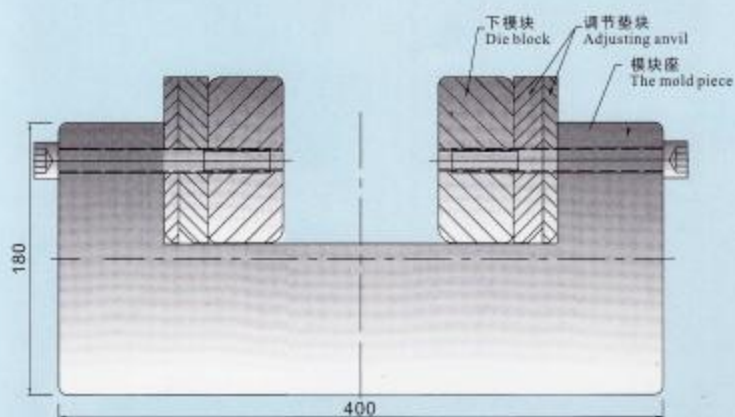
可调下模组合 Adjustable die assembly
